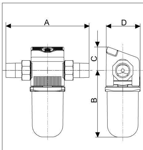
Illustration 2: Cotes de montage MHF mV
